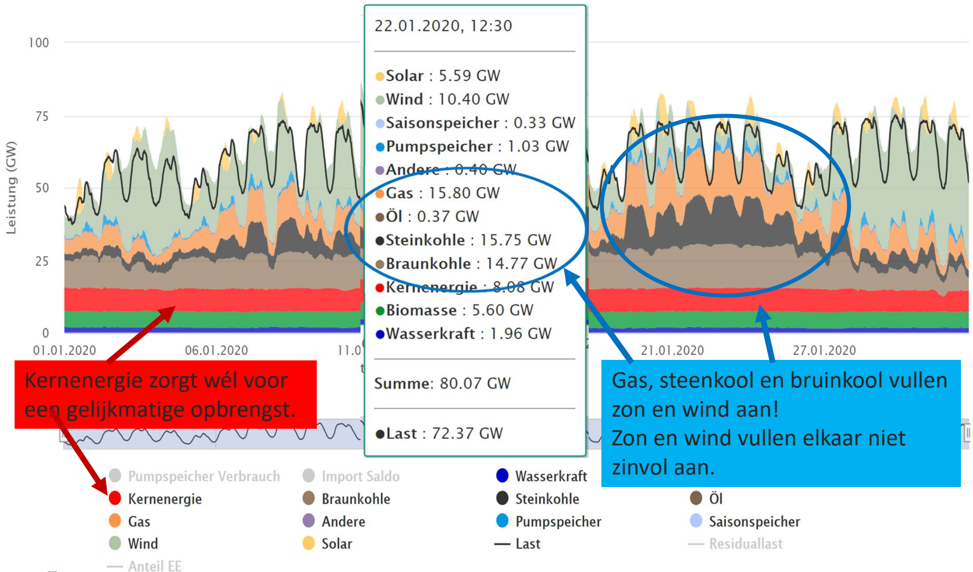
Stromerzeugung in Deutschland im Januar 2020
